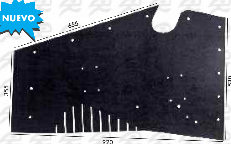
RCF 031 FALDILLA VIBRADOR TRASERO RT 65
